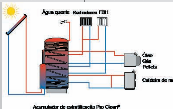
Acumulador de estratificação Pro-Clean®
